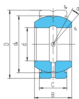
GEZ...ES-2RS
