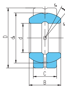
GEZ...ES
