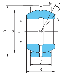
GEZ...ES-2RS
