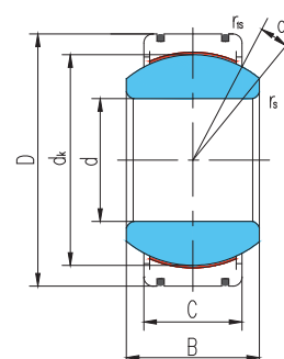
GE...XTL-2RS
